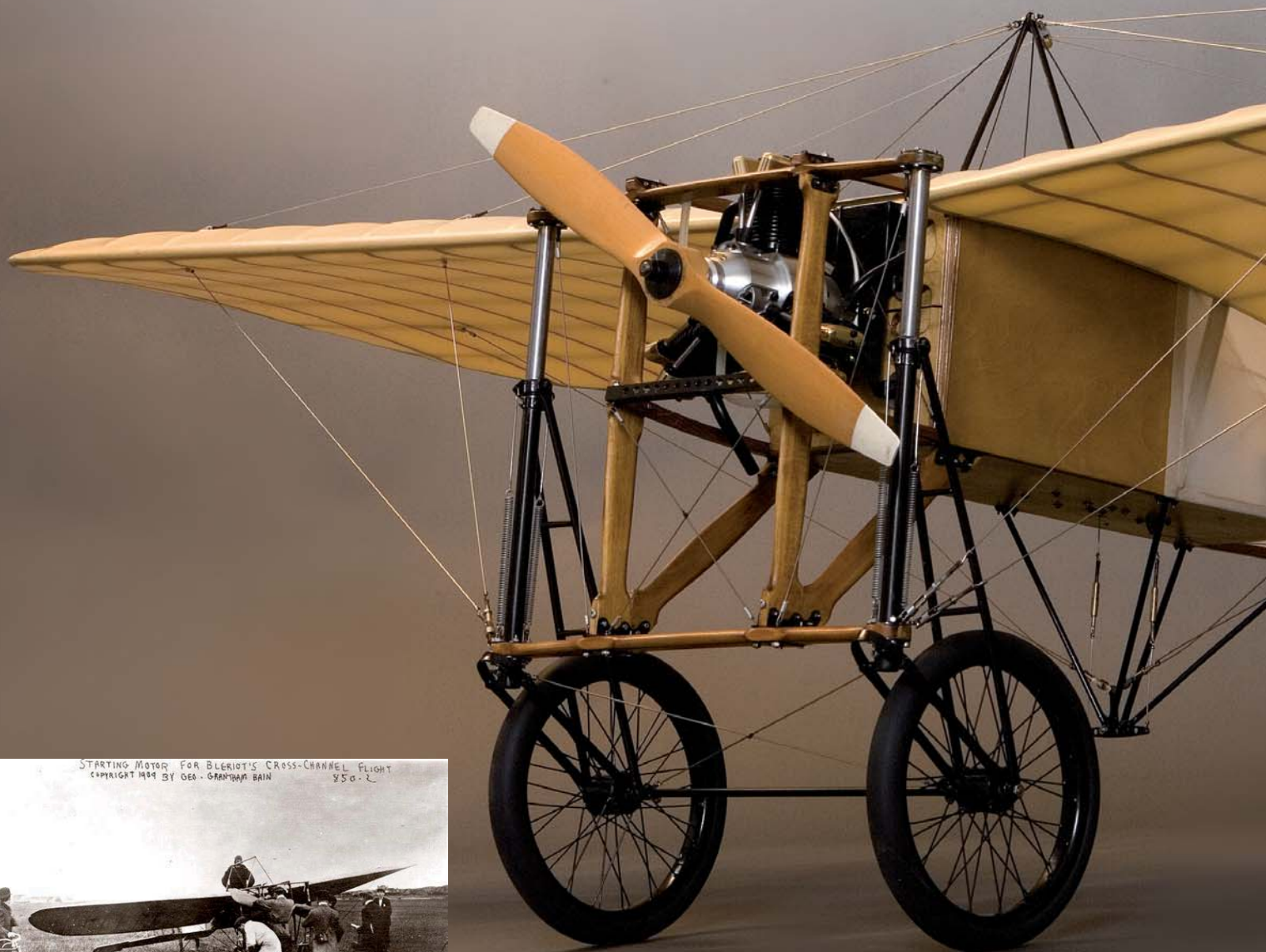
Foto a fianco: avviamento del Blériot prima della traversata della Manica. Nelle foto di fronte: motore Anzani ds 25 hp e Louis Blériot con Alessandro Anzani progettista e costruttore del motore. Il motore della trasvolata era un 3 cilindri a W, in seguito Anzani costruì anche motori a 3 cilindri a stella come quello utilizzato sul modello.
